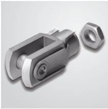
9440068987 SG-M20X1,5 Rod clevis
