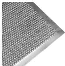
9491531987 Trieur Sheet Metal 1000*2000*2mm Ø 5.5
