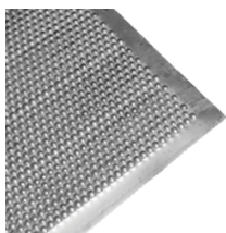
9491531987 Trieur Sheet Metal 1000*2000*2mm Ø 11
